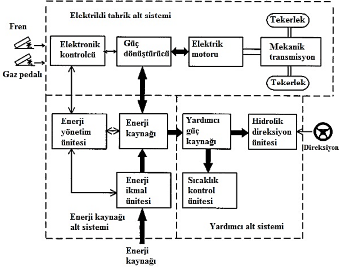
Şekil 2.16. Hibrit araçlardaki enerji yönetim sisteminin diğer ünitelerle haberleşmesini gösteren diyagram (Chan, 2002)
