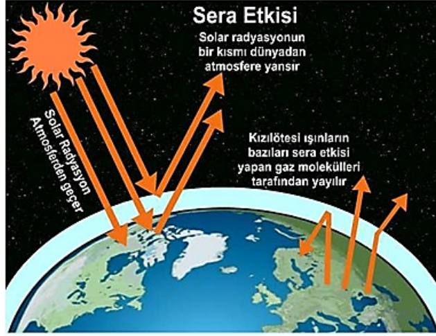
Şekil 1.10. Sera etkisi (Çelik ve ark.,2008)
