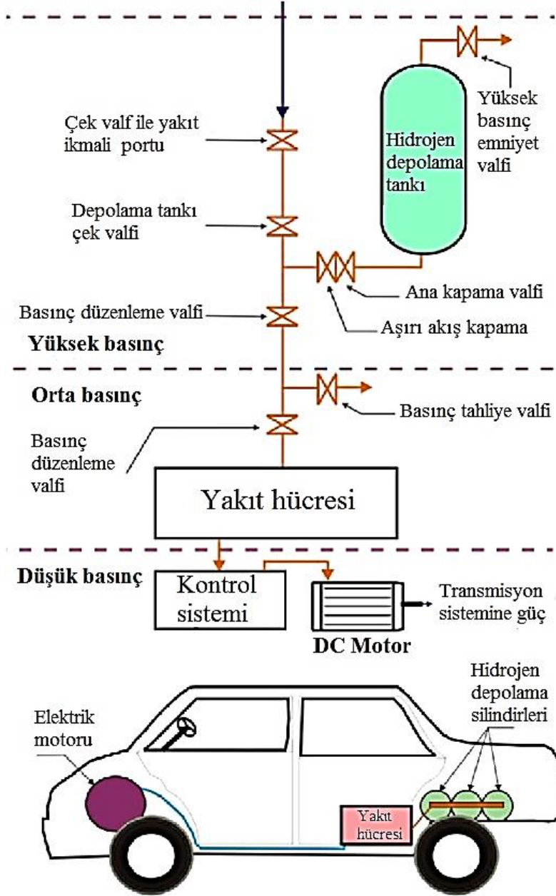
Şekil 3.3. Yakıt hücreli araçların dahili hidrojen depolama aşamaları (Salvi ve Subramanian, 2015)
