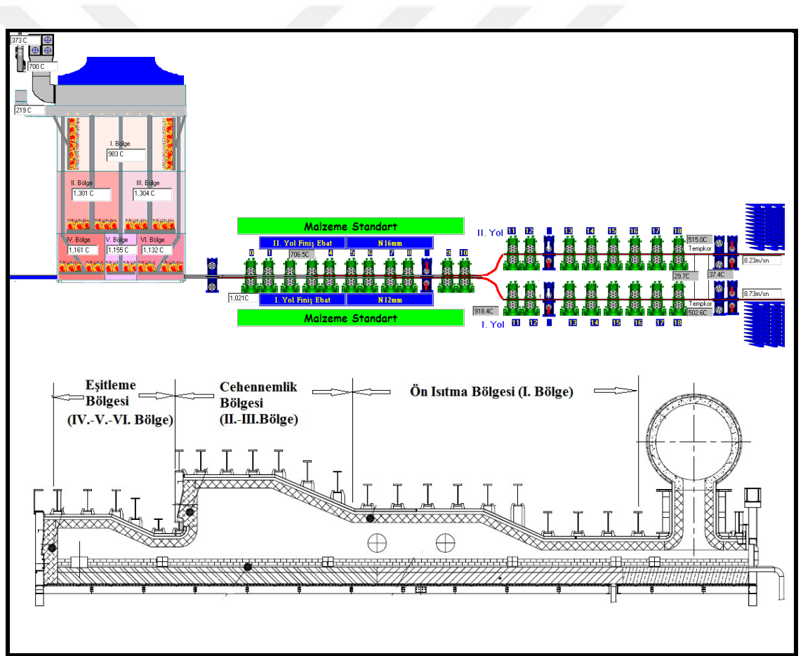
Şekil 3.3. Tav Fırını ve haddeleme prosesi şematik görüntüsü
