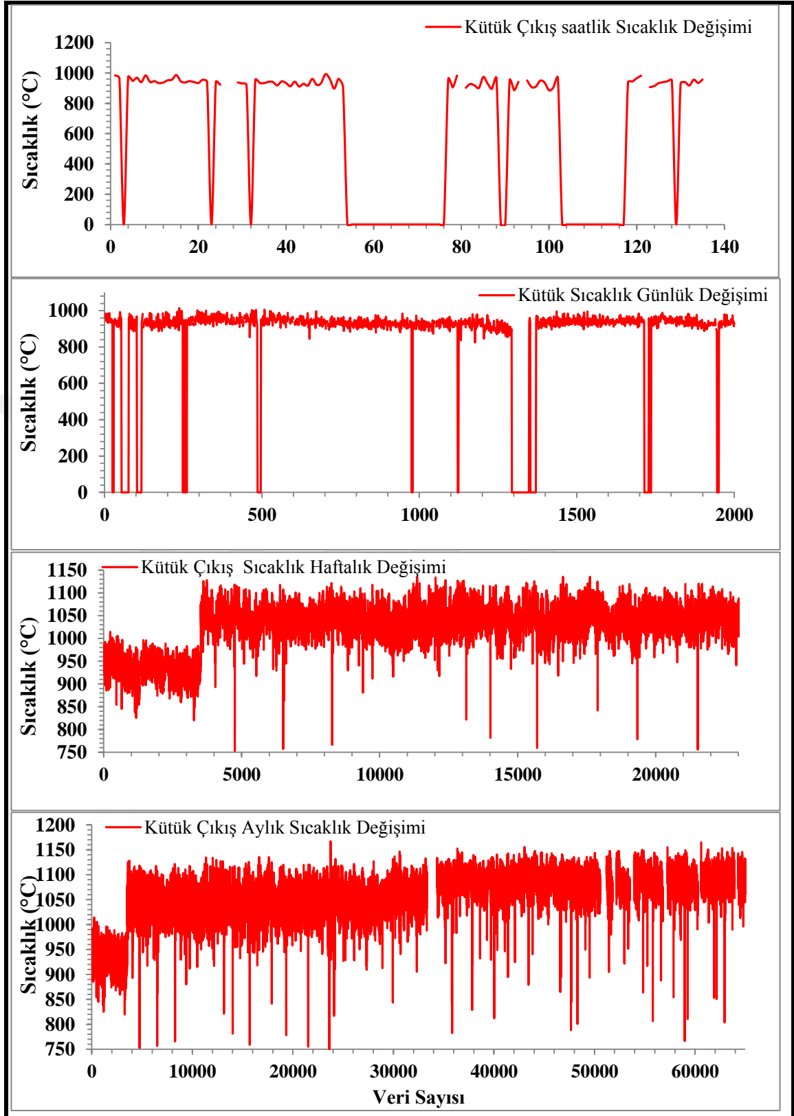
Şekil 4.2. Tav Fırınındaki kütük çıkış sıcaklık değişimleri
